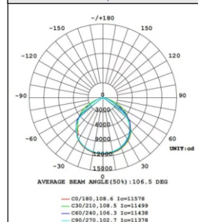
Curva fotométrica(Photometric Curve)
