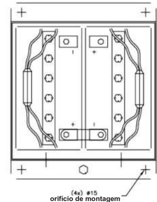
VISTA DO PLANO DO BANCO DE BATERIAS
