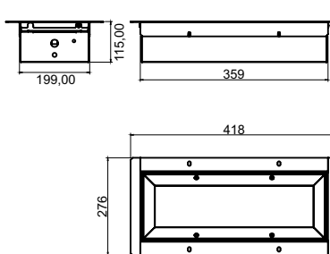
Suporte Embutir (EB)
