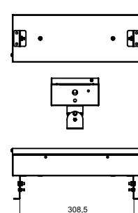
Suporte Teto Angular (TA)
