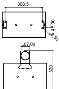
Suporte Poste (PO)
