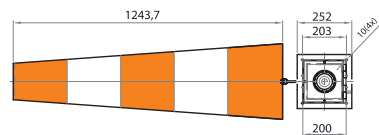
VISTA SUPERIOR ( SOMENTE LUMINÁRIA DE OBSTRUÇÃO) UPPER VIEW (ONLY OBSTRUCTION LUMINAIRE) SEM ESCALA/UNSCALED
