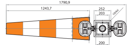
VISTA SUPERIOR ( OPÇÃO 2 PROJETORES) OVERVIEW (OPTION 2 FLOODLIGHTS) SEM ESCALA/UNSCALED
