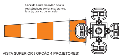
VISTA SUPERIOR ( OPÇÃO 4 PROJETORES) OVERVIEW (OPTION 4 FLOODLIGHTS) SEM ESCALA/UNSCALED
